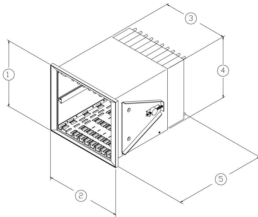
Установочные размеры мини-стойки 3500 для монтажа на панели
